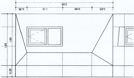
แบบขยายผนังด้าน TypeB-B ด้านหน้า มาตราส่วน 1 : 25
