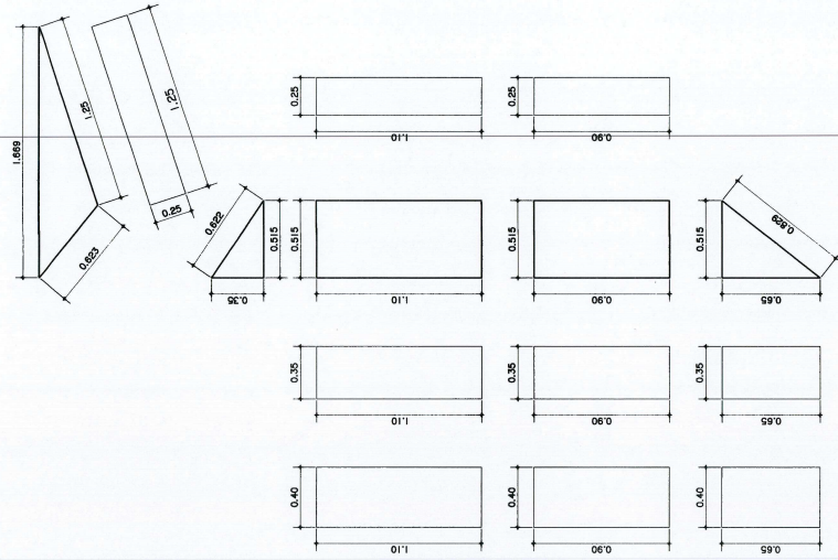
แบบขยายผนัง TypeB-B มาตราส่วน 1 : 25
