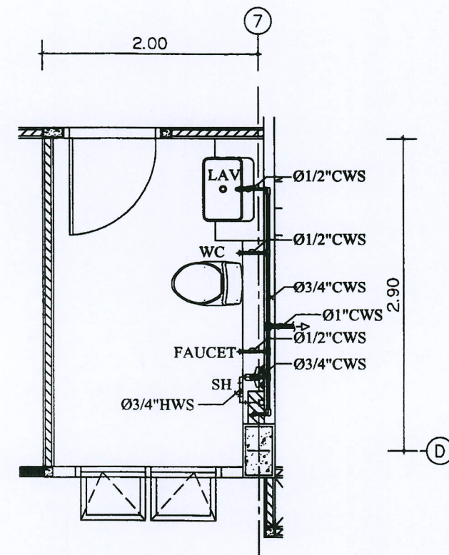
แบบขยายการเดินท่อน้ำ CWS ภายในห้องน้ำ WC-01 มาตราส่วน 1 : 50
