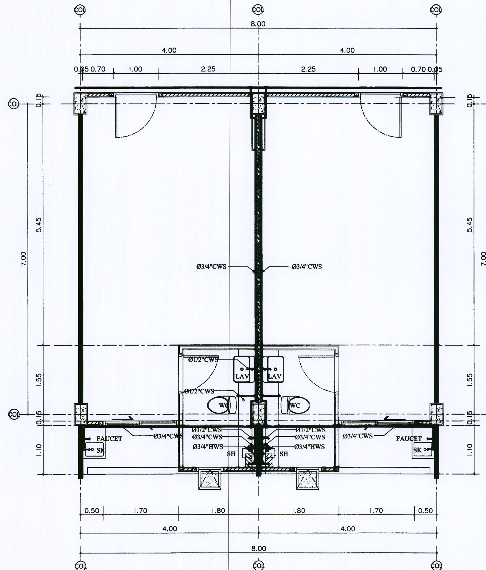
แบบขยายการเดินท่อน้ำ CWS ภายในห้องน้ำ WC-04 มาตราส่วน 1 : 50
