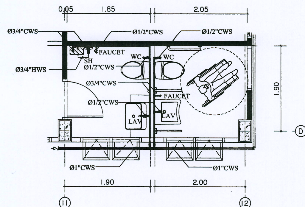
แบบขยายการเดินท่อน้ำ CWS ภายในห้องน้ำ WC-02, WC-03 มาตราส่วน 1 : 50
