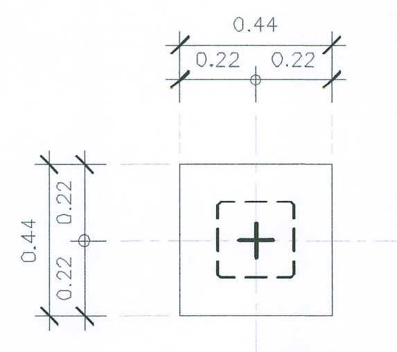
PLAN F122 SCALE 1:25
