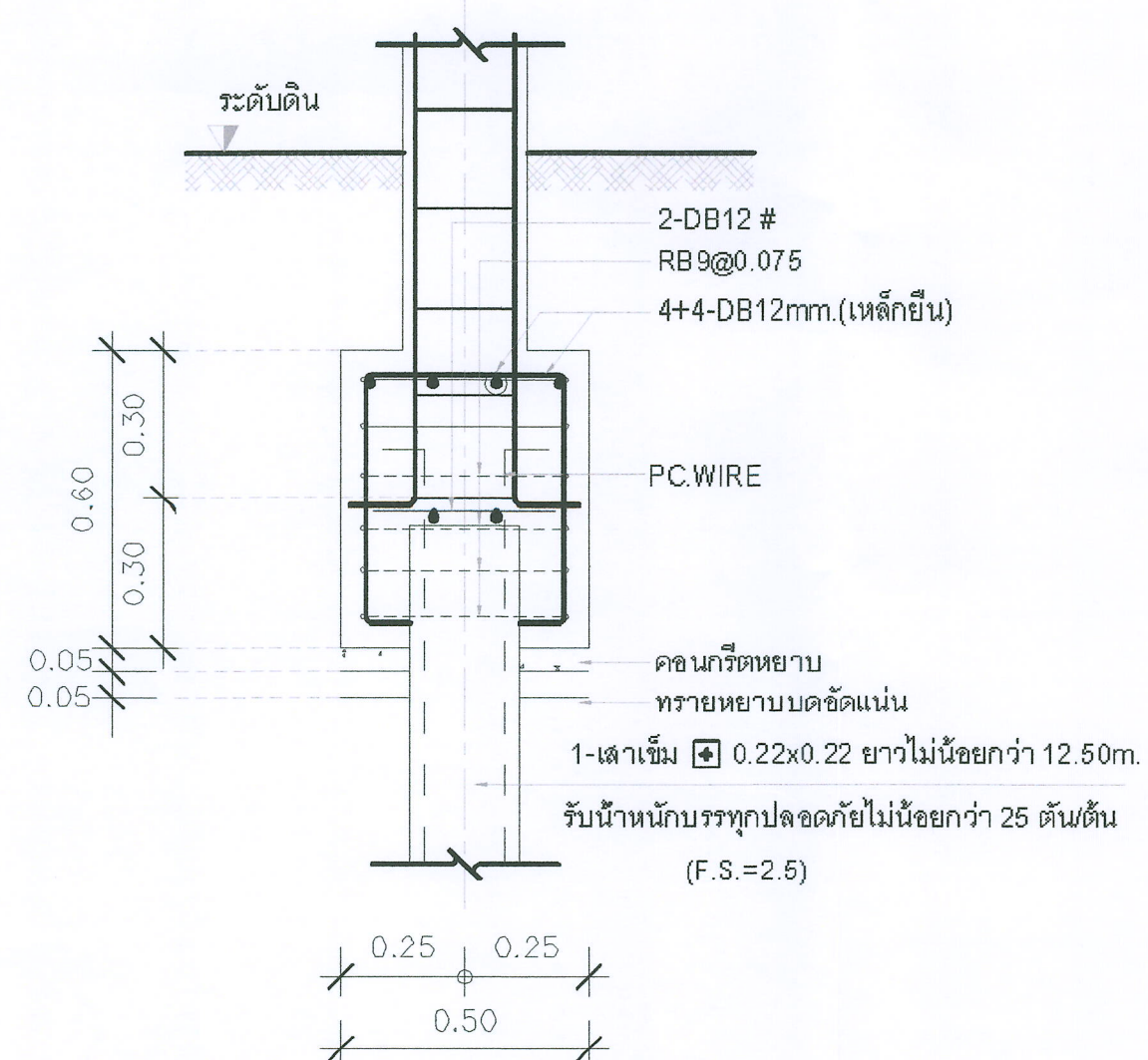
SECTION F122 SCALE 1:25
