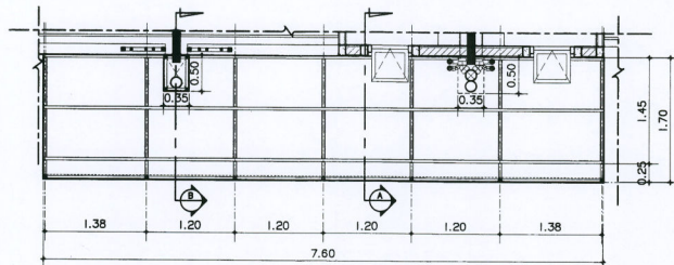
แบบขยายหลังคาทางเข้า ผังโครงสร้างหลังคา มาตราส่วน 1 : 50
