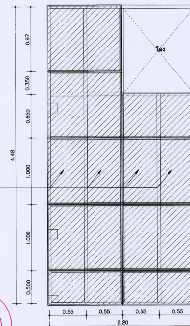
DT-ST4 แบบขยายหลังคานบันได AST-06 มาตรฐาน 1 : 25
