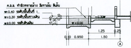
แบบขยายบันได ST-04_รูปตัด D มาตราส่วน 1 : 50
