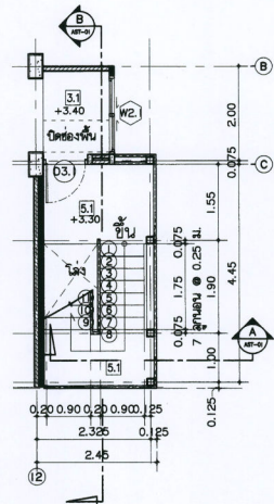
แบบขยายบันได ST-02 ฝั่งพื้น ชั้นที่ 2 มาตราส่วน 1 : 75
