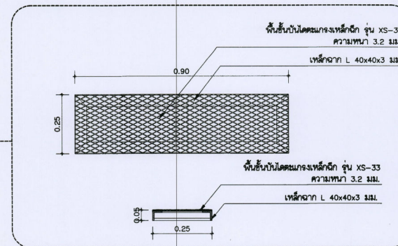
แบบขยายขั้นบันได มาตรฐาน 1 : 10
