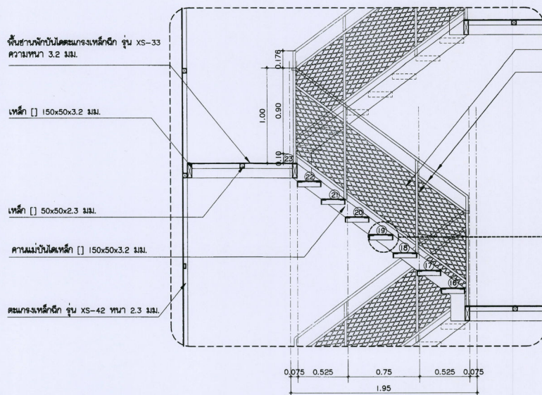
DT-ST2 แบบขยายบันได AST-06 มาตรฐาน 1 : 25
