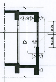
แบบขยายผนัง 02-รูปตัด A มาตราส่วน 1 : 50
