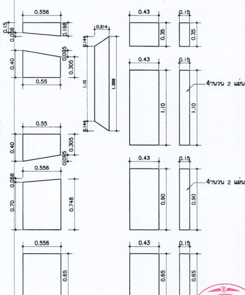
แบบขยายผนัง Type A-A มาตราส่วน 1 : 25
