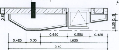
แบบขยายผนังคาน Type A-A ผนัง มาตราส่วน 1 : 25
