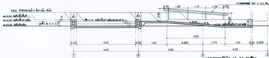
แบบขยายบันได ST-04_รูปตัด A มาตราส่วน 1 : 50
