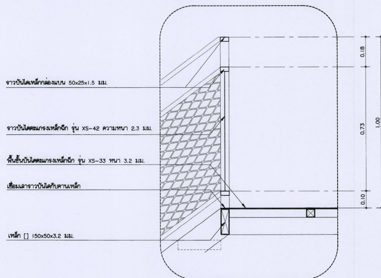
DT-ST3 แบบขยายราวบันได AST-06 มาตรฐาน 1 : 25
