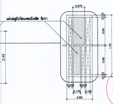
DT-02 AD-03 แบบขยายผนัง 02 มาตราส่วน 1 : 50
