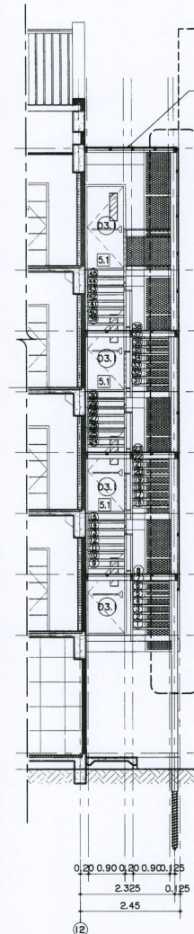
แบบขยายบันได ST-02-รูปตัด A มาตราส่วน 1 : 75
