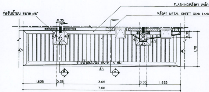
แบบขยายหลังคาทางเข้า ผังพื้น มาตราส่วน 1 : 50
