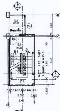
แบบขยายบันได ST-02 ฝั่งพื้น ชั้นที่ 4 มาตราส่วน 1 : 75
