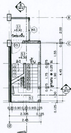
แบบขยายบันได ST-02 ฝั่งพื้น ชั้นที่ 3 มาตราส่วน 1 : 75
