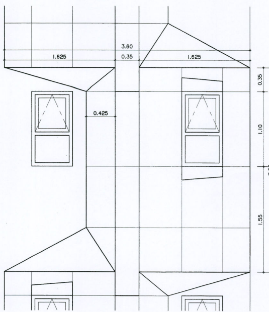
แบบขยายผนังคาน Type A-A ฐาน มาตราส่วน 1 : 25
