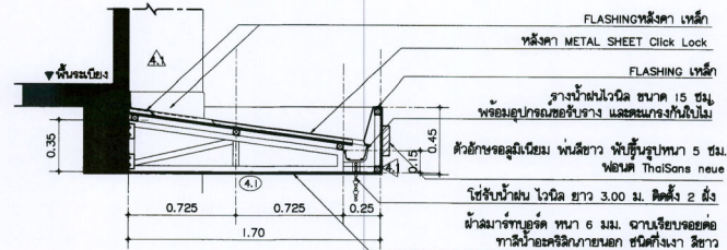
แบบขยายหลังคาทางเข้า รูปตัด A มาตราส่วน 1 : 25
