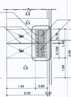
แบบขยายผนัง 02-รูปด้าน มาตราส่วน 1 : 50
