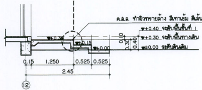
แบบขยายบันได ST-05_รูปตัด A มาตราส่วน 1 : 50
