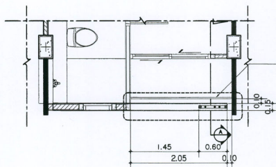
แบบขยายผนัง 02-ผนัง มาตราส่วน 1 : 50
