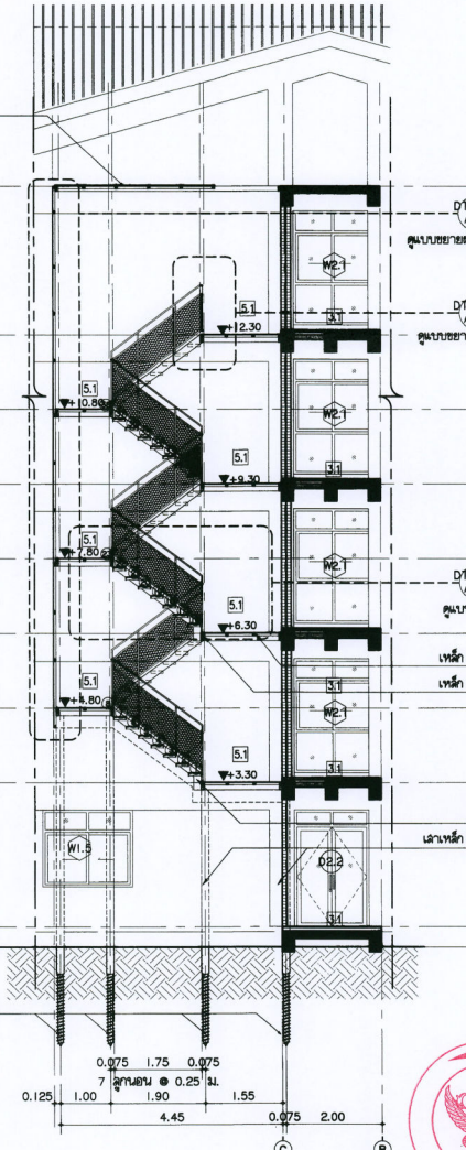
แบบขยายบันได ST-02-รูปตัด B มาตราส่วน 1 : 75
