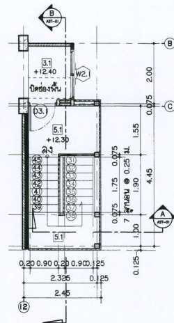
แบบขยายบันได ST-02 ฝั่งพื้น ชั้นที่ 5 มาตราส่วน 1 : 75
