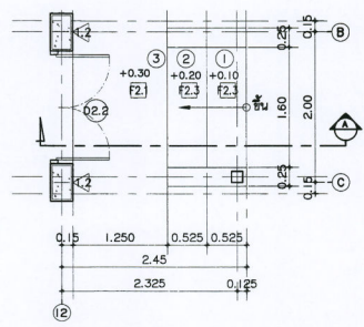
แบบขยายบันได ST-05_ผังพื้น มาตราส่วน 1 : 50
