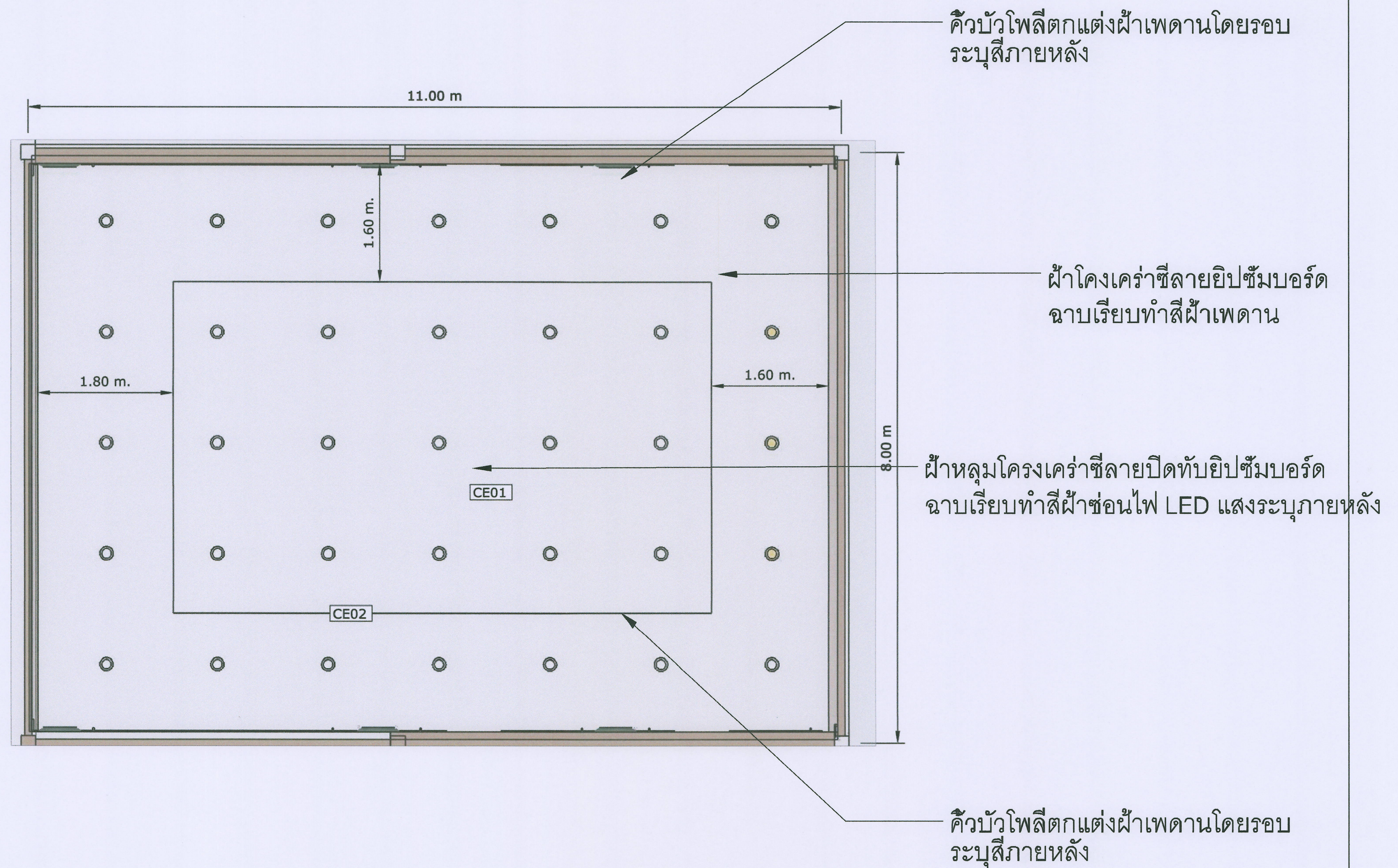
แปลนฝ้าเพดานห้องประชุม 20 ที่นั่ง ชั้น 2
