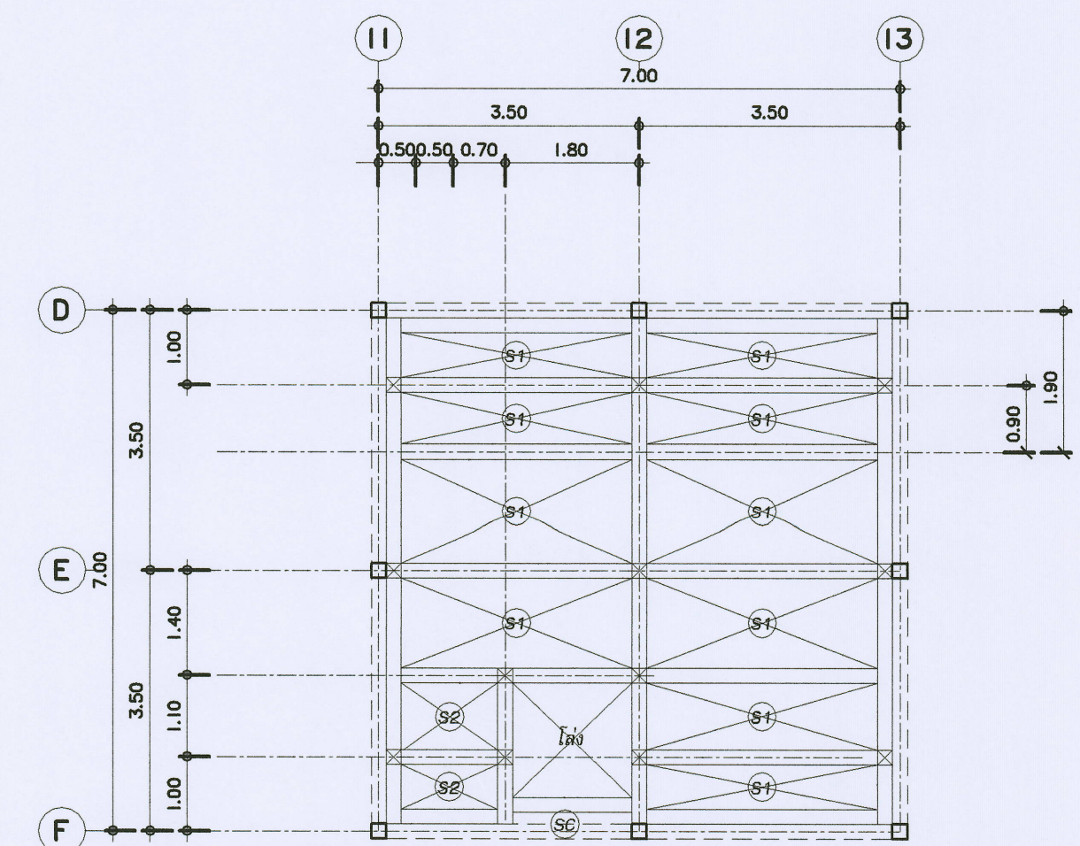
แบบแปลนพื้น เสา ห้องน้ำชั้น 2 มาตราส่วน 1 : 50
