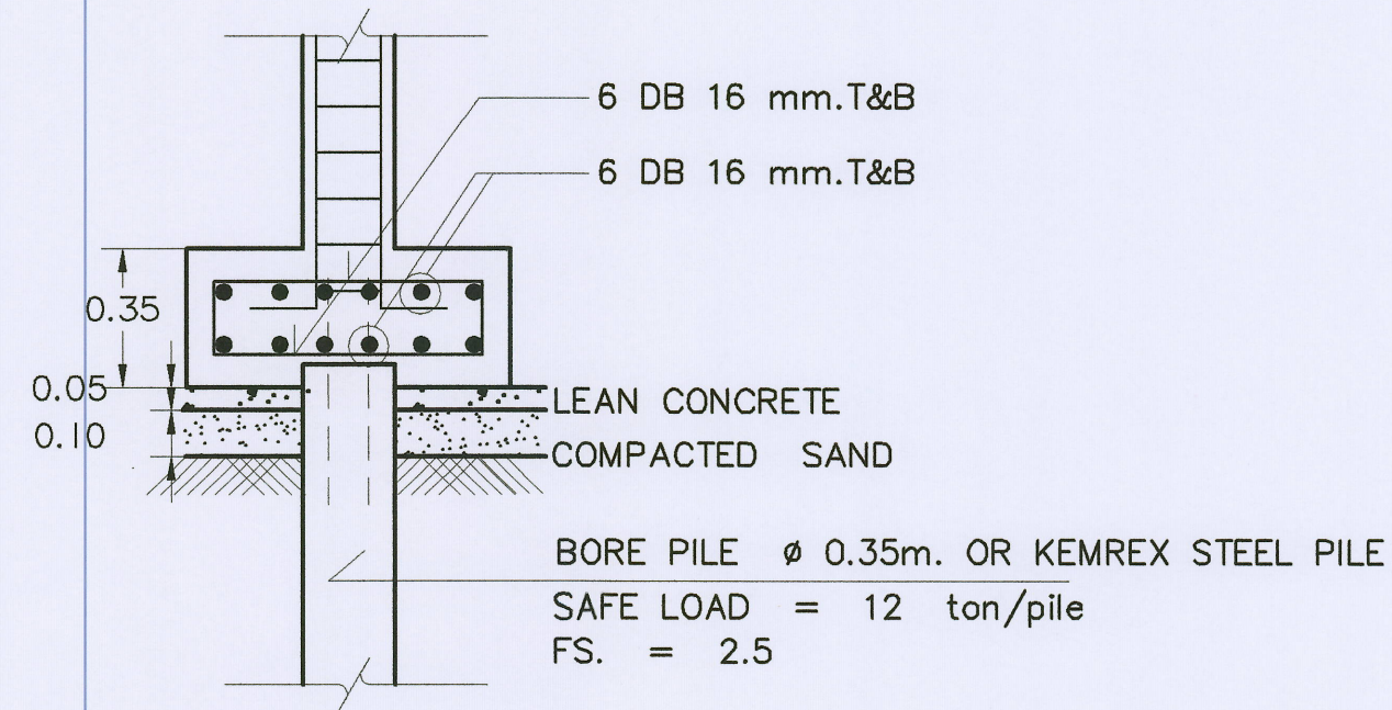
FOOTING F1 SCALE -
