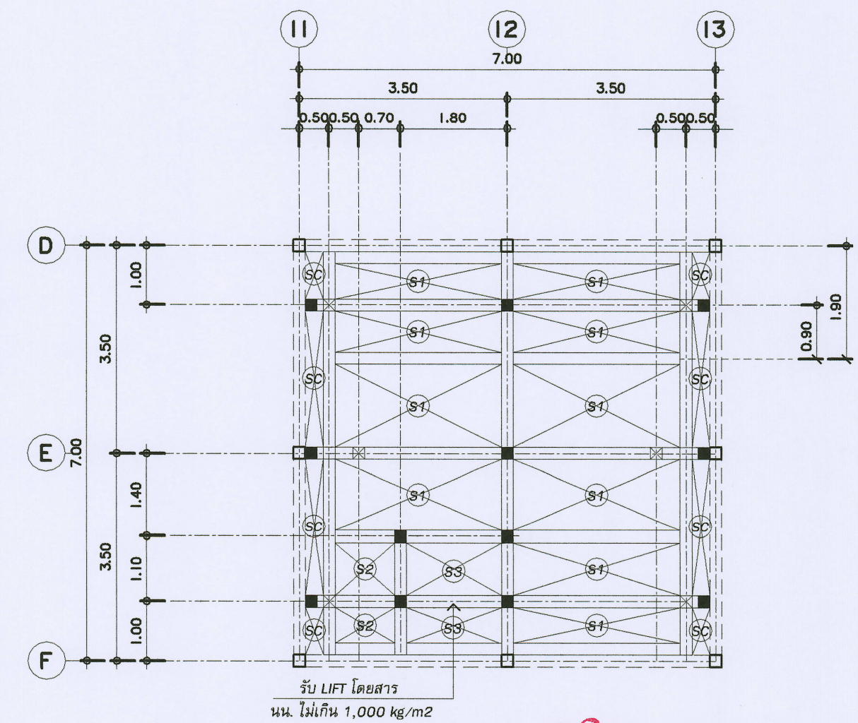
แบบแปลนพื้น เสา ห้องน้ำชั้น 1 มาตราส่วน 1 : 50
