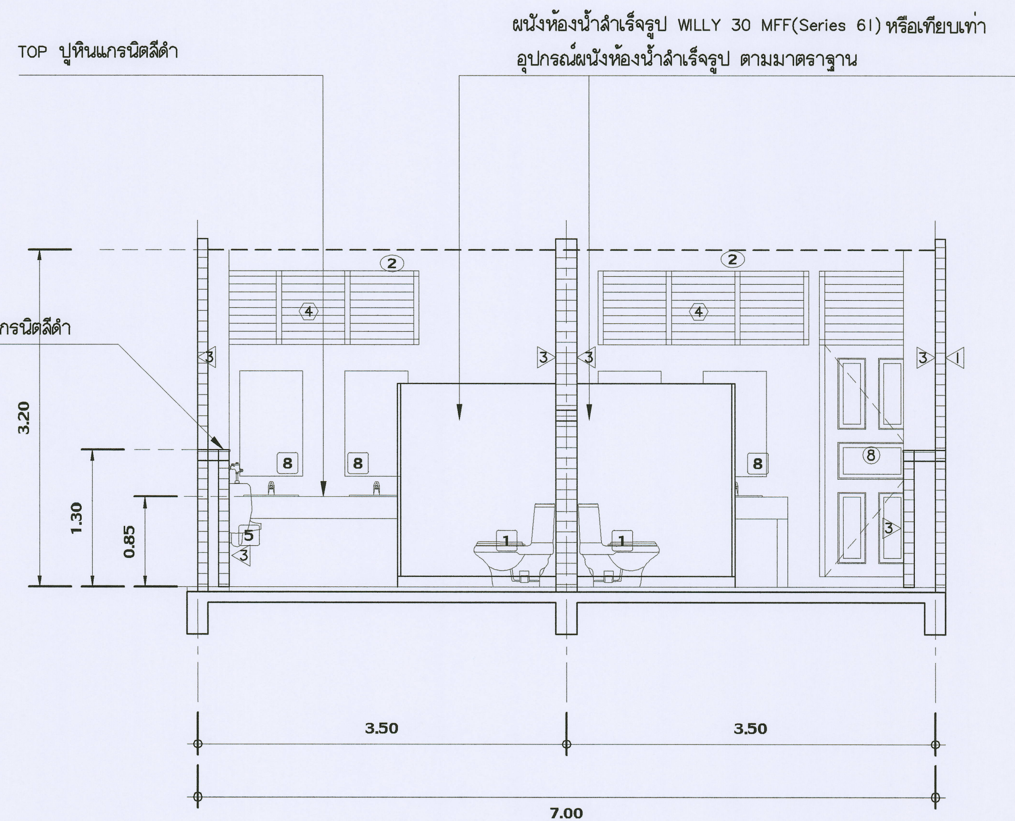
แบบแสดง ขยายรูปตัดห้องน้ำ มาตราส่วน 1 : 25
