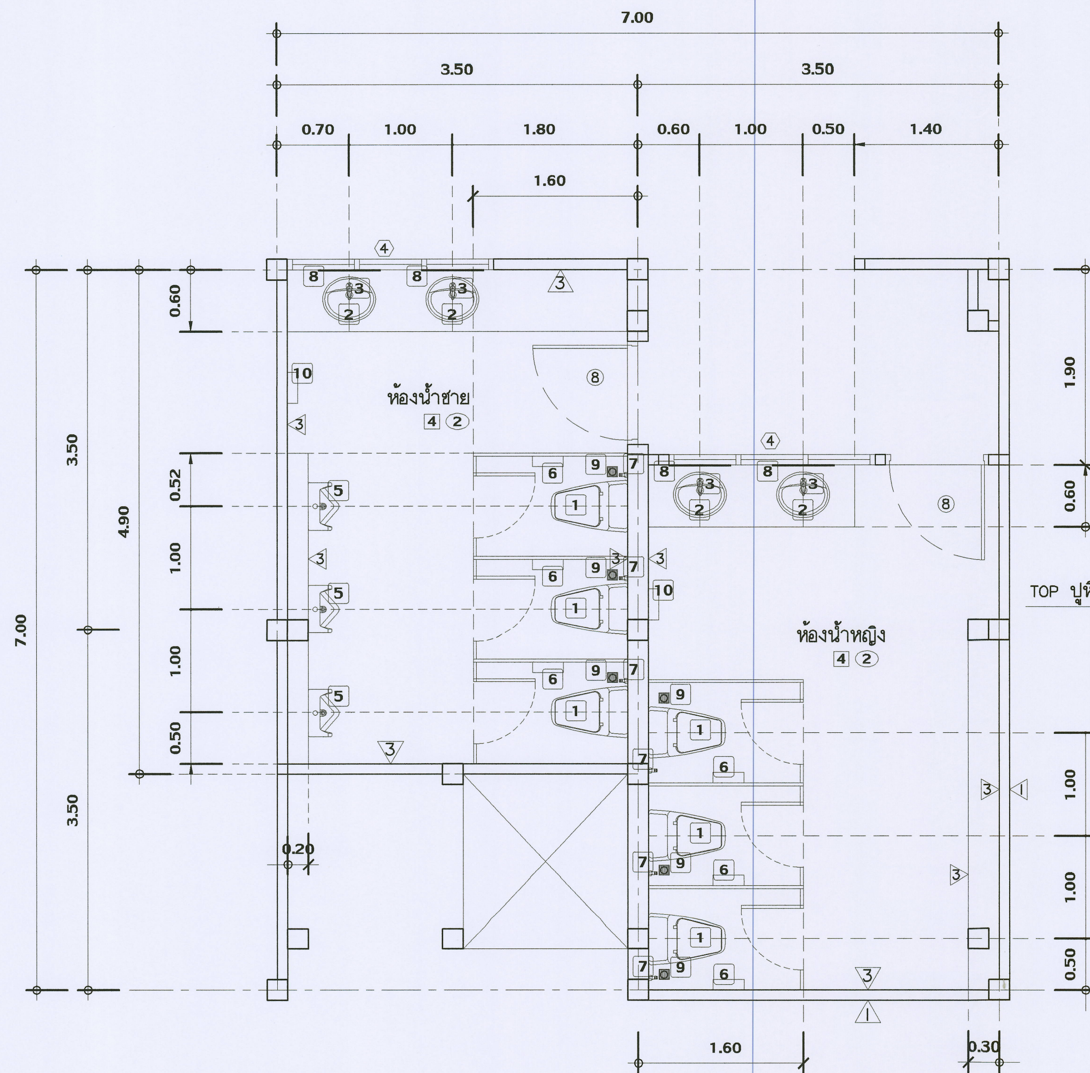
แบบแสดง แปลนขยายห้องน้ำ มาตราส่วน 1 : 25
