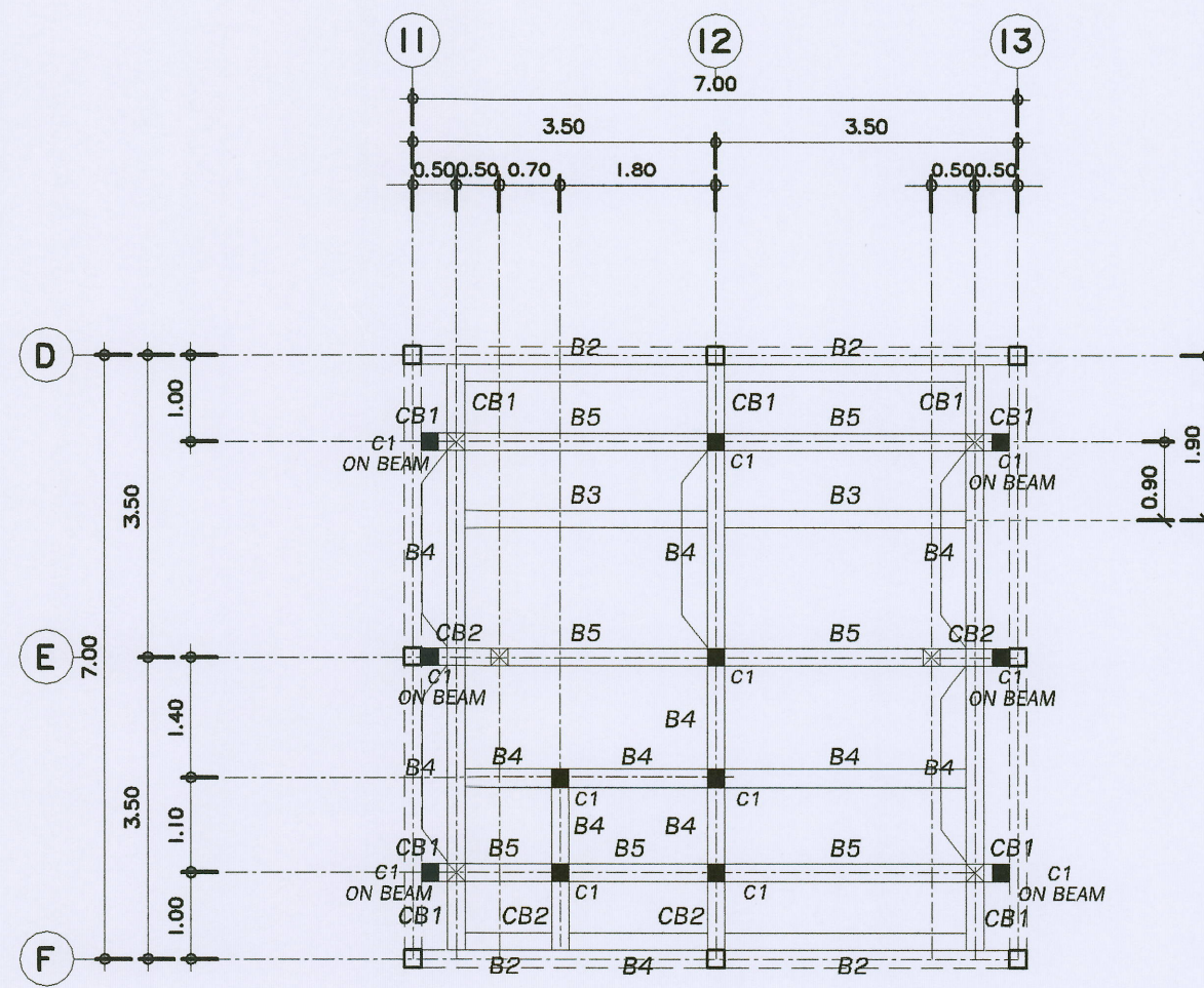
แบบแปลนคานา ห้องน้ำชั้น 1 มาตราส่วน 1 : 50
