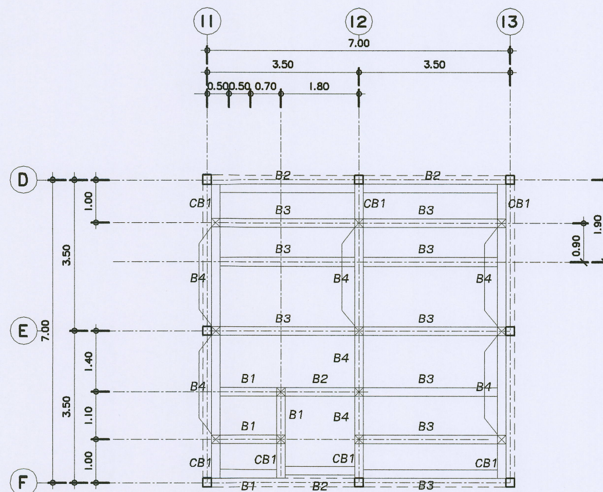
แบบแปลนคานา ห้องน้ำชั้น 2 มาตราส่วน 1 : 50
