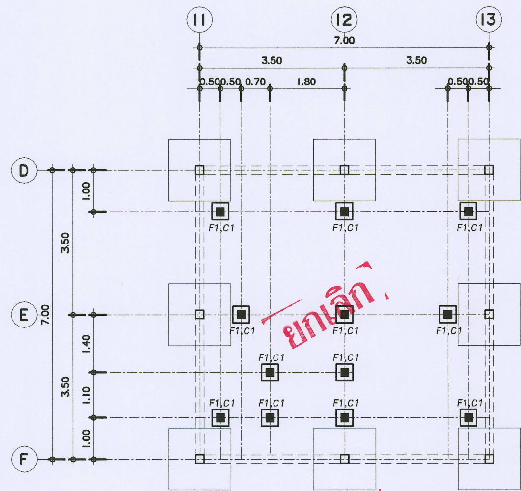
แบบแปลนฐานราก ห้องน้ำชั้น 1 มาตราส่วน 1 : 50
