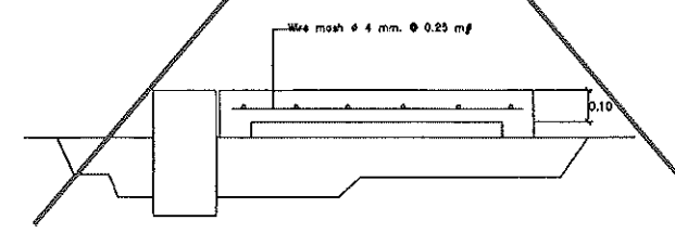
ขยายพื้น GS-01 SCALE 1:25
