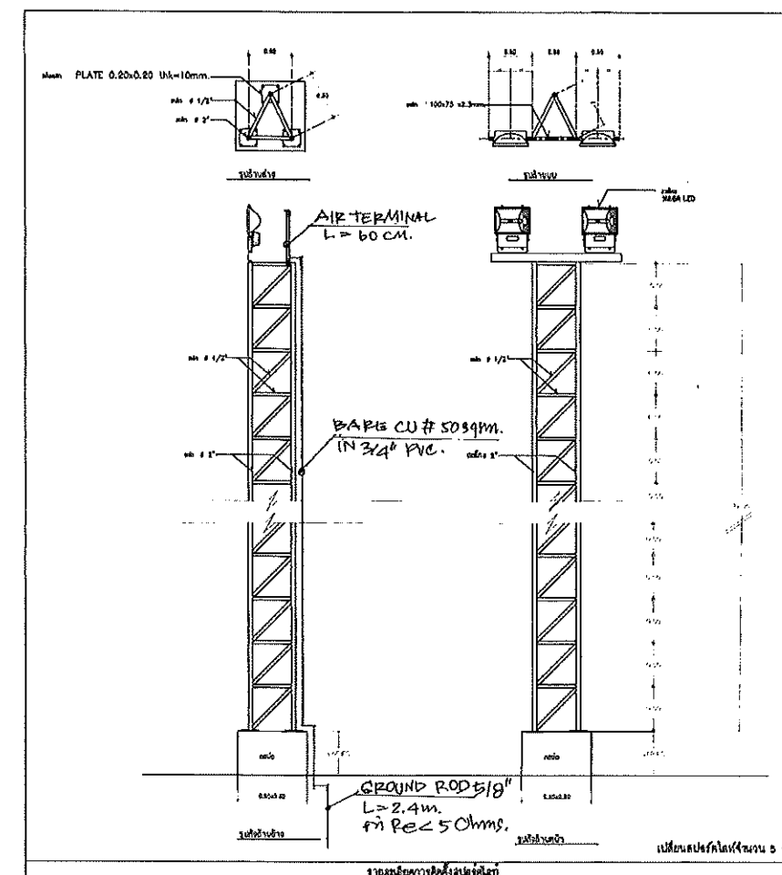
การติดตั้งเสาหลอดไฟ
