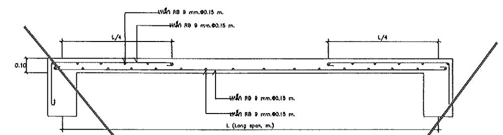
ขยายพื้น S-01 SCALE 1:25
