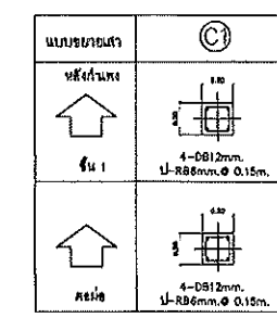
แบบขยายเสา มาตราส่วน
