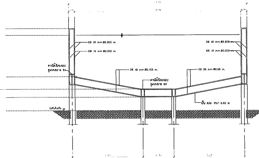
โครงสร้างถังตกตะกอน SCALE 1:100
