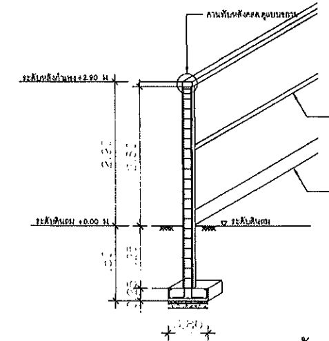
รูปตัดรั้วกำแพง มาตราส่วน
