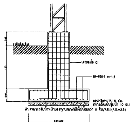
แบบขยายฐานรากเสาหลอดไฟ
