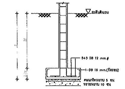
แบบขยายฐานราก มาตราส่วน
