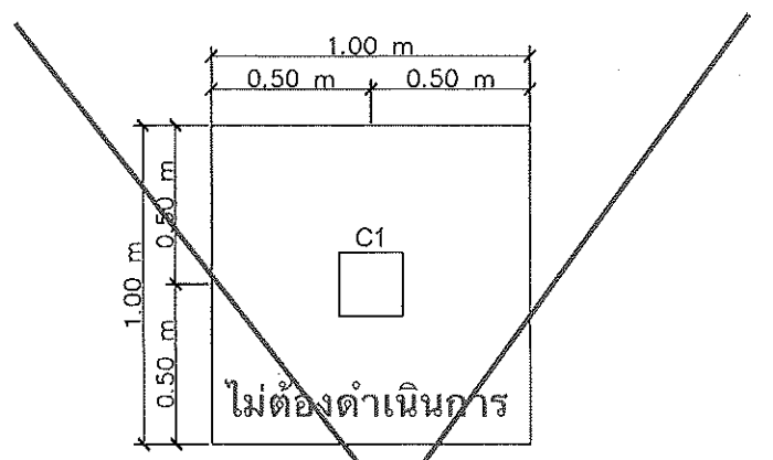
ขยายพื้น GS-01 SCALE 1:25
