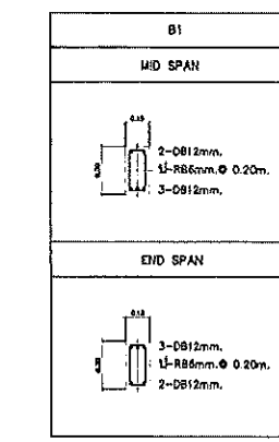
แบบขยายคาน มาตราส่วน
