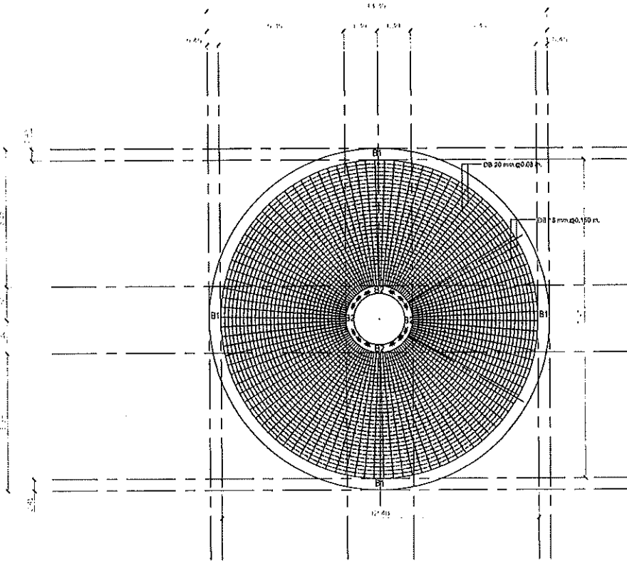
แปลนการเสริมเหล็กพื้นถังตกตะกอน SCALE 1:100
