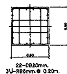
แบบขยายคอกม่อเสาหลอดไฟ
