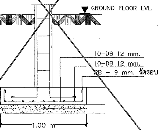
ขยายฐานราก SCALE 1:25
