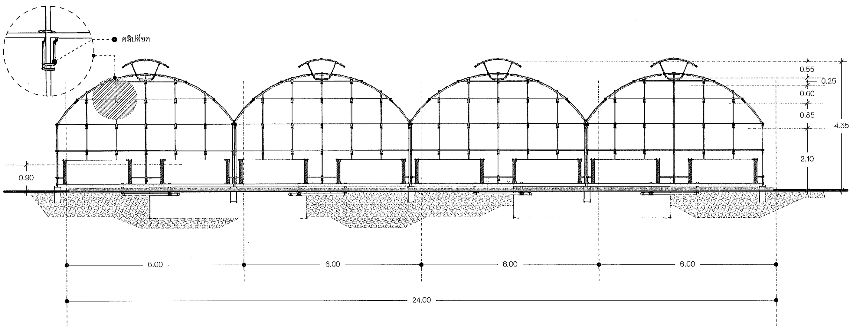
แบบรูป ตัด A1-A1 Scale 1 : 75
