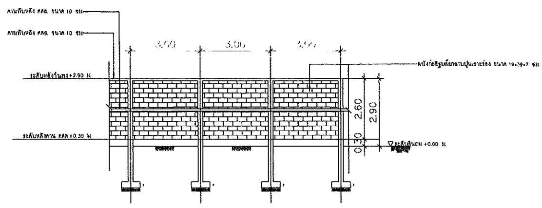
แบบด้านรั้ว มาตราส่วน
