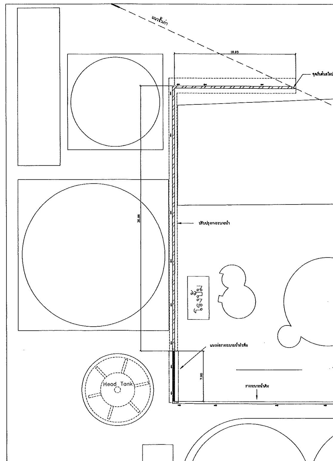
แปลนปรับปรุงและก่อสร้างรางระบายน้ำเพิ่มเติม SCALE 1:150
