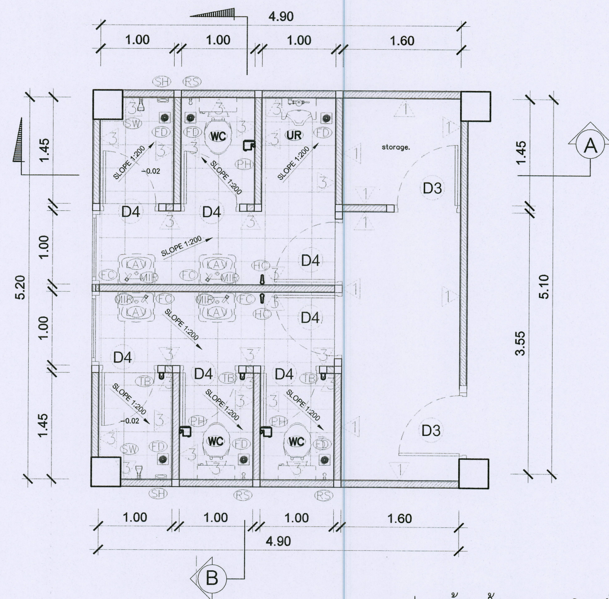
แปลนห้องน้ำชาย-หญิง ชั้น 1
