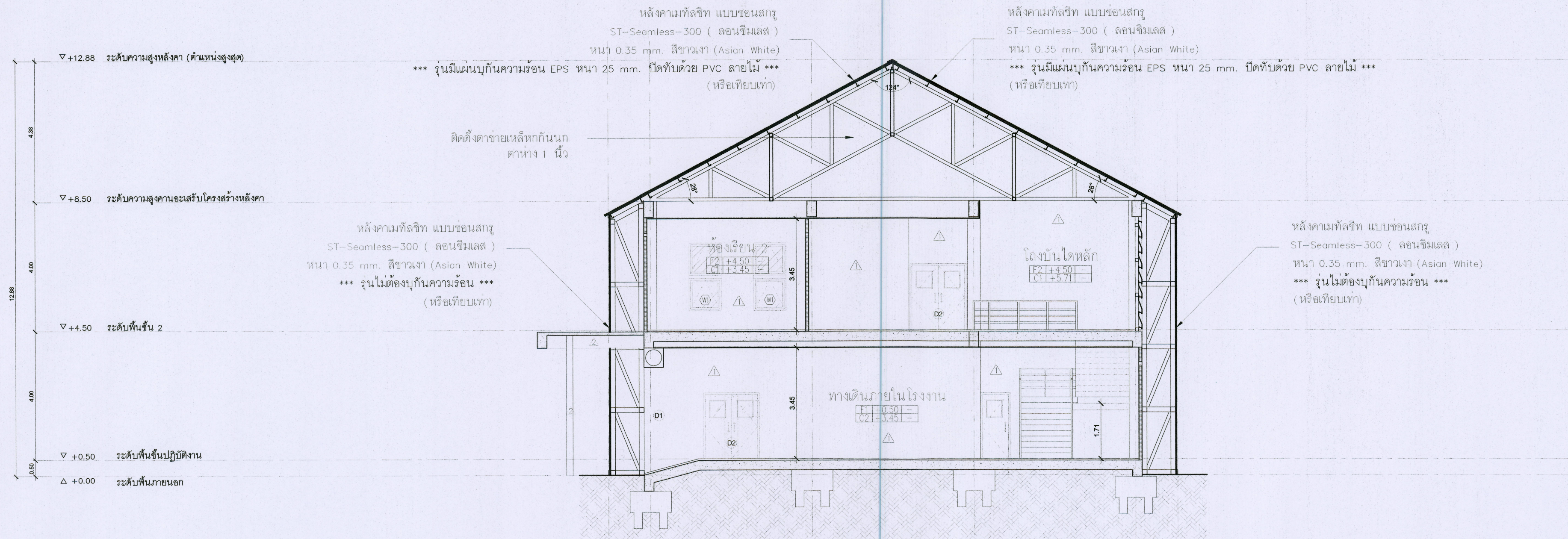
รูปตัด A-A
