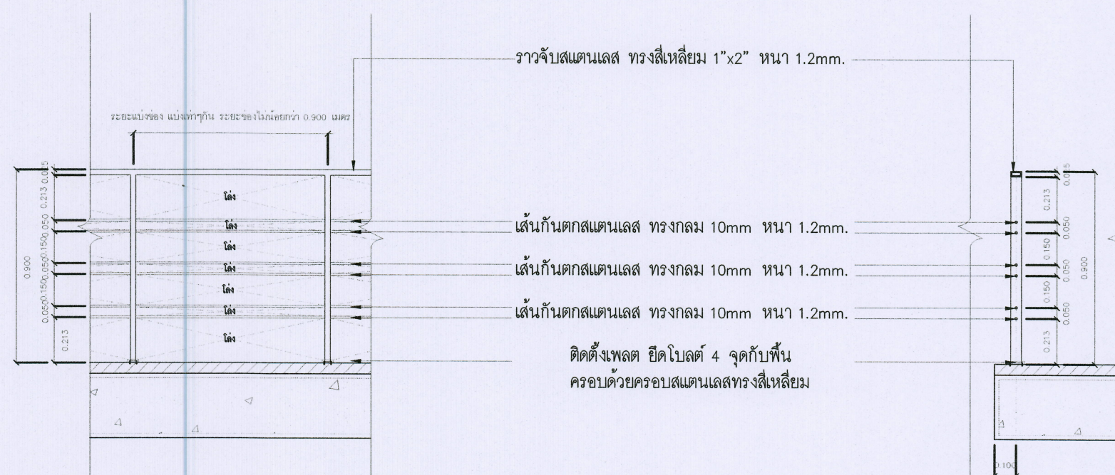
รูปด้าน
