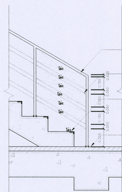
รูปตัด
