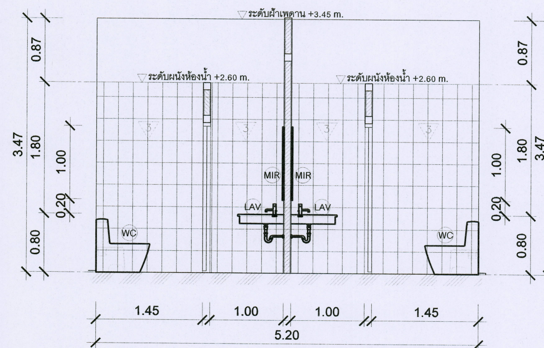
รูปตัดห้องน้ำชาย-หญิง B-B
