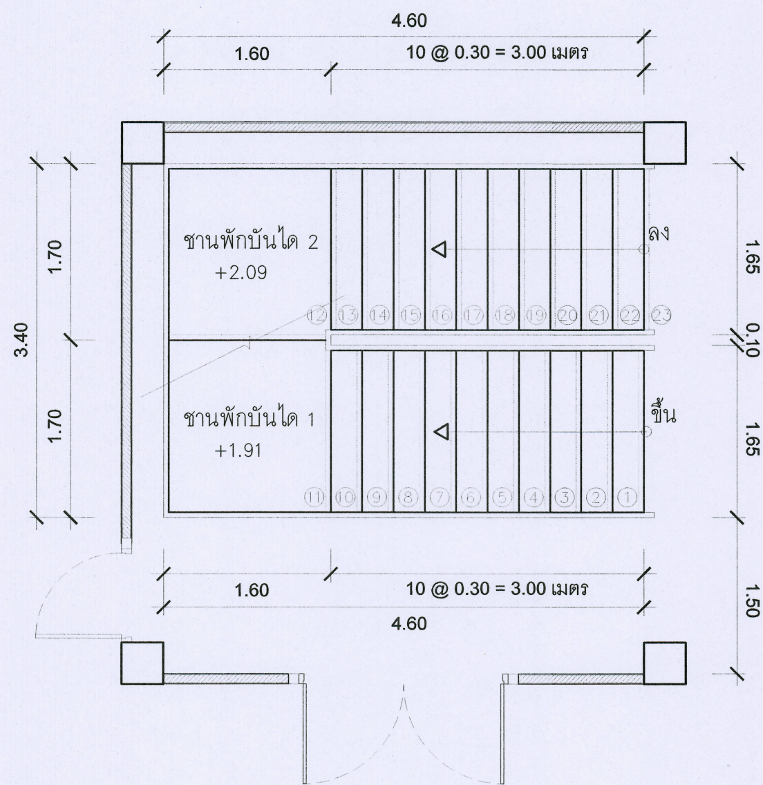
แปลนขยายบันไดหลัก
